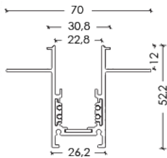
Afmetingen in mm Dimensions en mm
