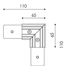
I L-90°hoek (mini)
