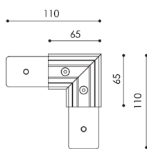
I L-90°hoek (surface)
